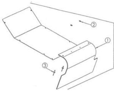
ET - Nr. 7236 Bodenplatte vollst.
