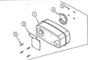
ET - Nr. 7227 Schalldämpfer vollst.
